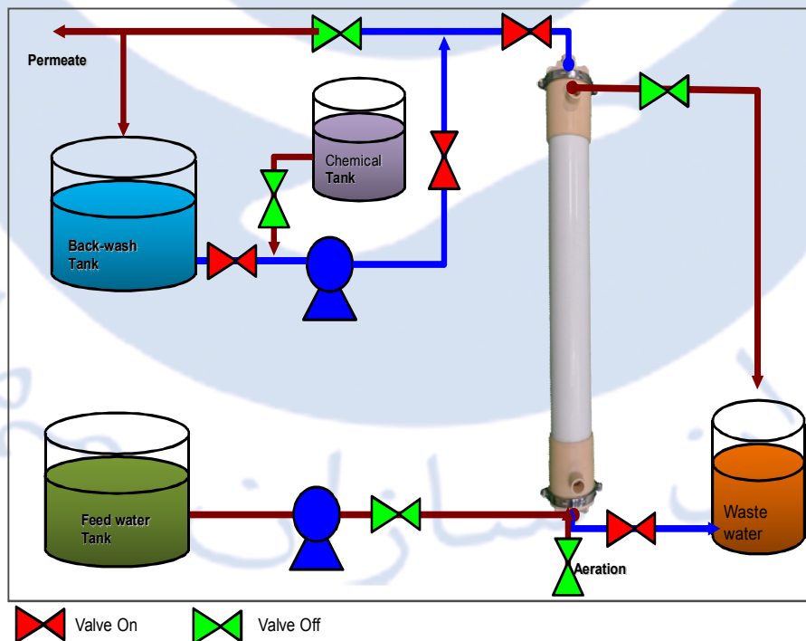
نمودار جریانی در حالت شست و شوی معکوس:
